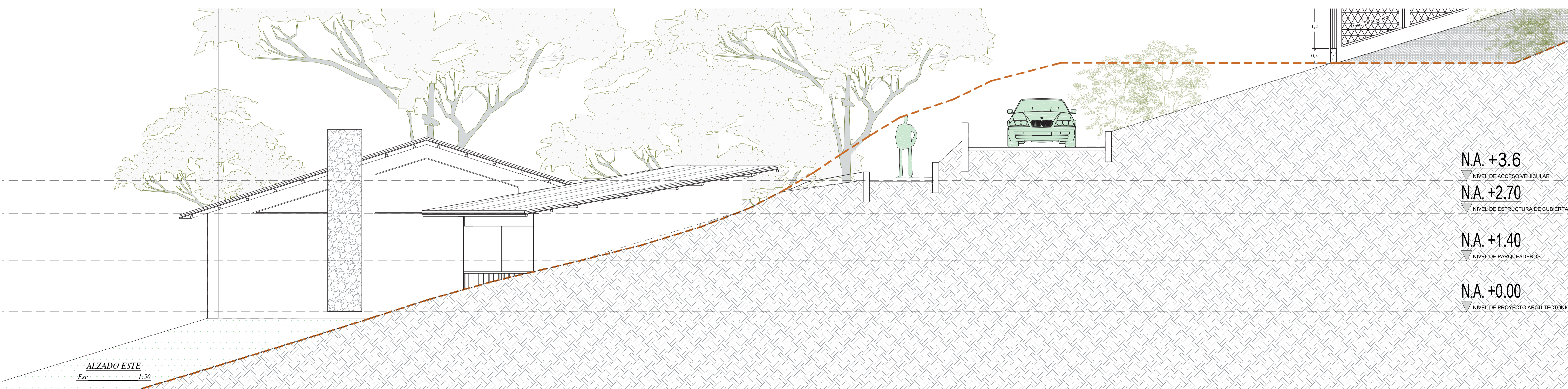
ALZADO OESTE Esc 1:50
