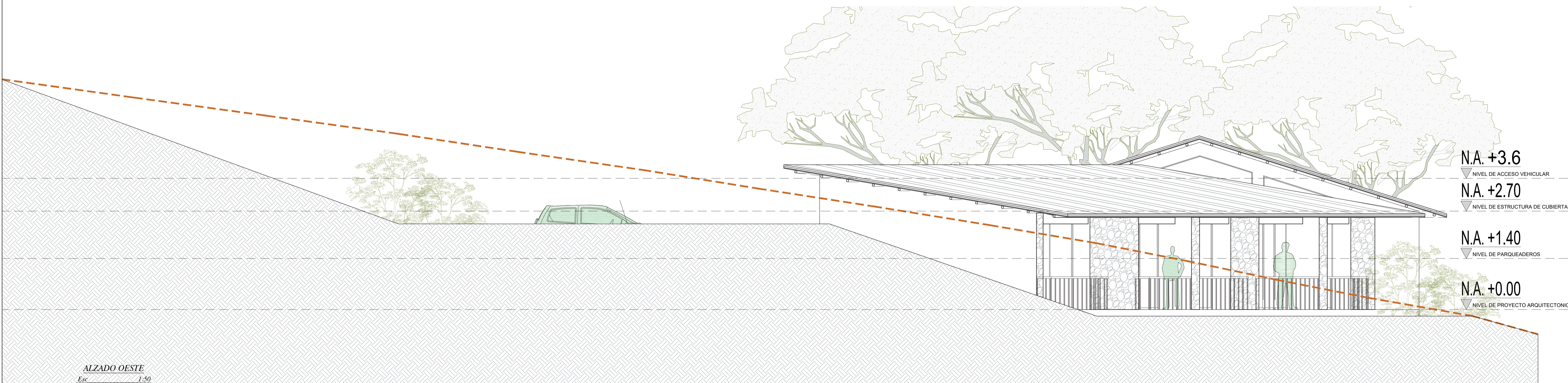
ALZADO SUR Esc 1:50
