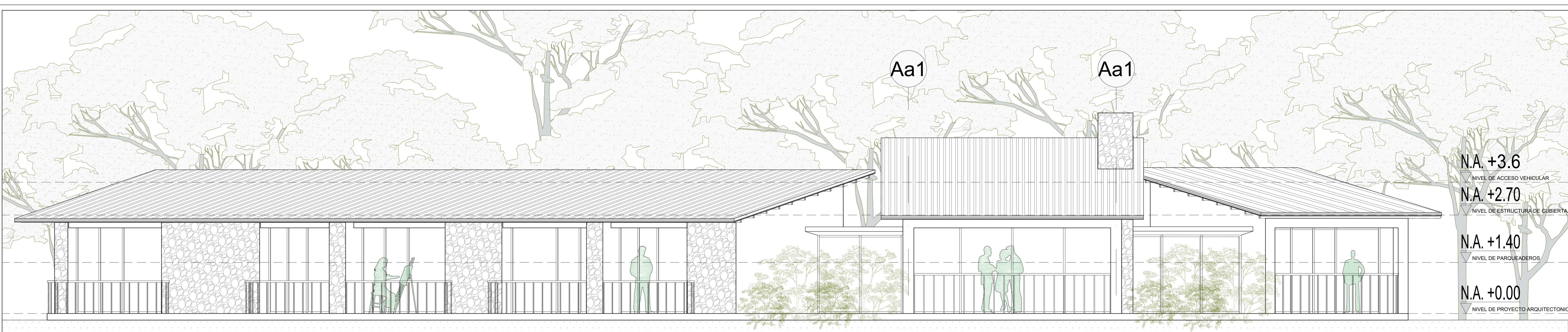
ALZADO SUR Esc 1:50
